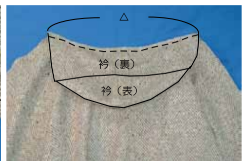
⑥ 衿を付ける 身頃と衿を中表に合わせて△印を縫い、縫代を下側に倒す
