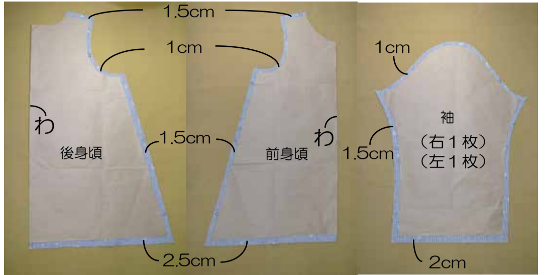
縫代の付け方 (参考)
